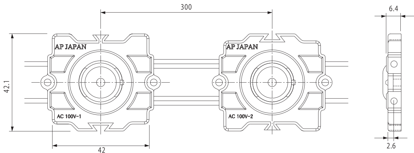
● 側面図
