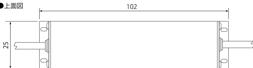
●上面図
