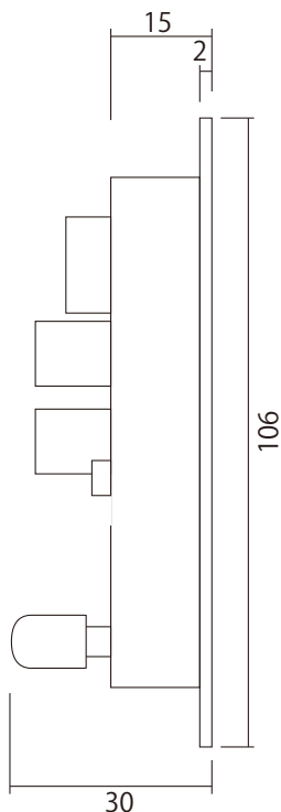
●側面図
