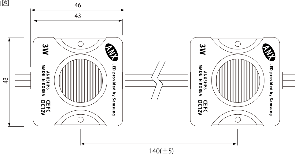
●リード線カット配置詳細
