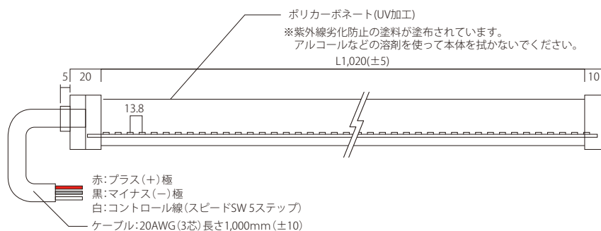
● 正面図
